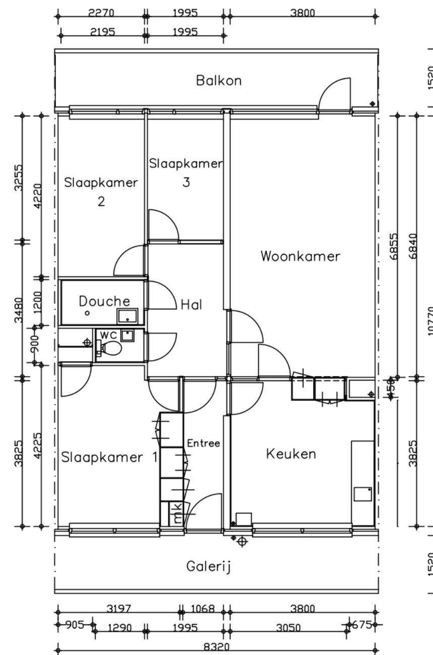
Verdieping 5
