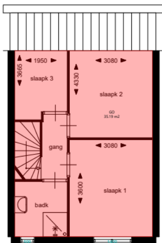
Verdieping_1e
