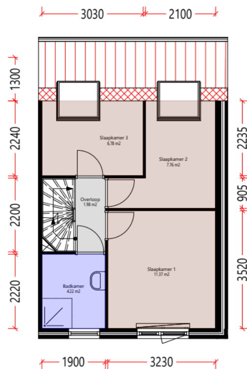
Verdieping_1e
