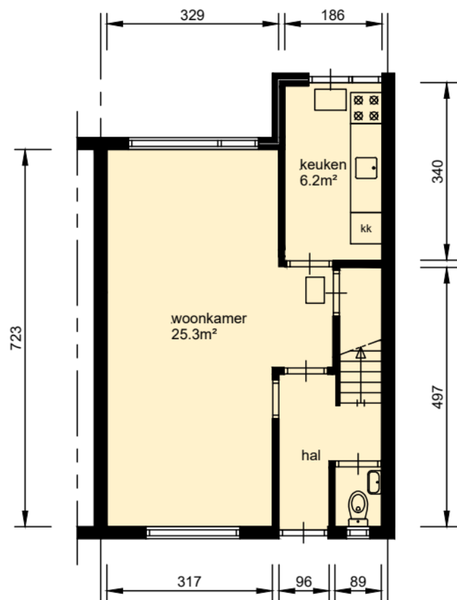
begane grond
