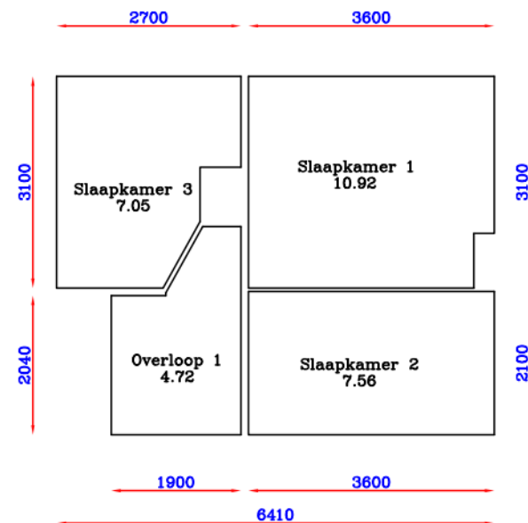
1e Verdieping
