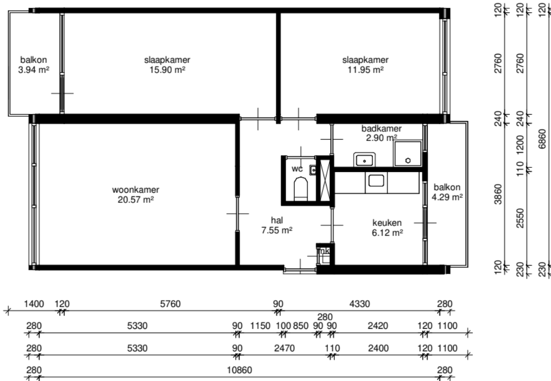
eerste verdieping
