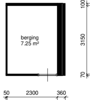
begane grond
