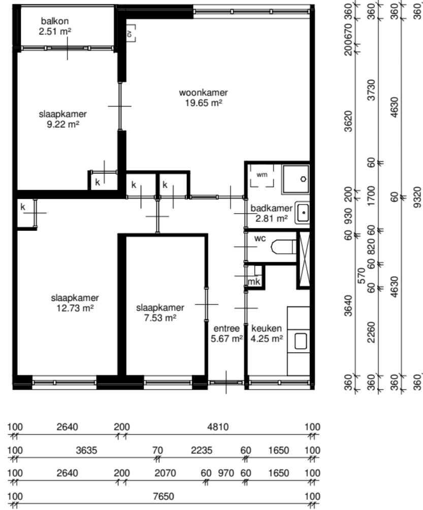
eerste verdieping
