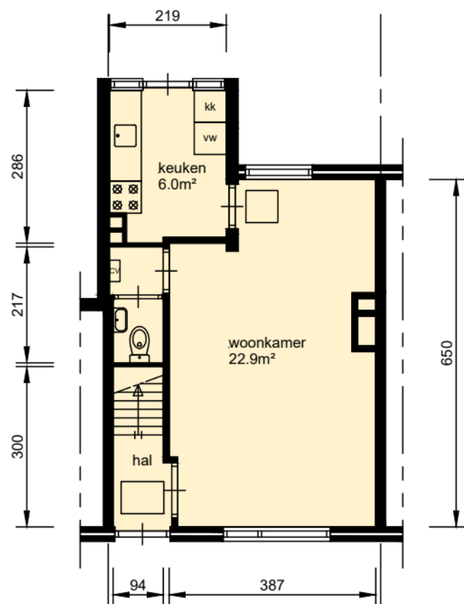
begane grond
