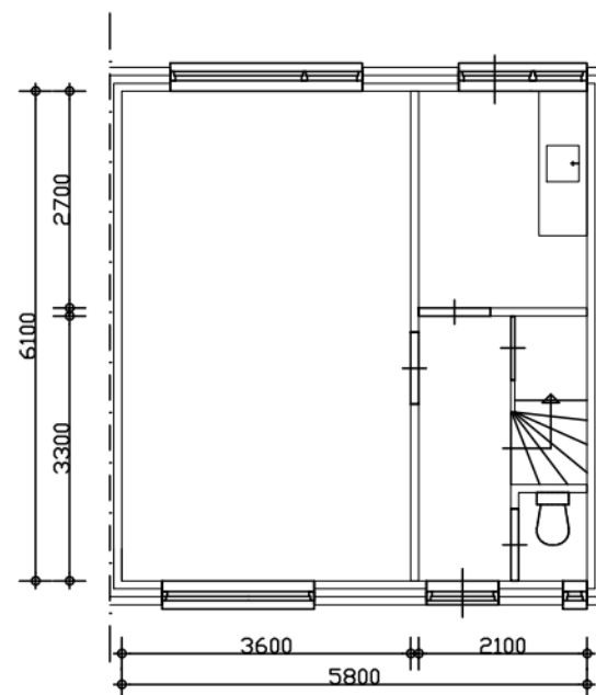
Beganegrond
