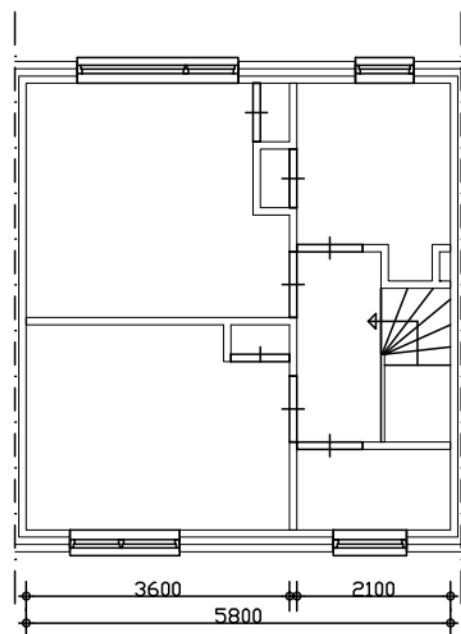
Verdieping
