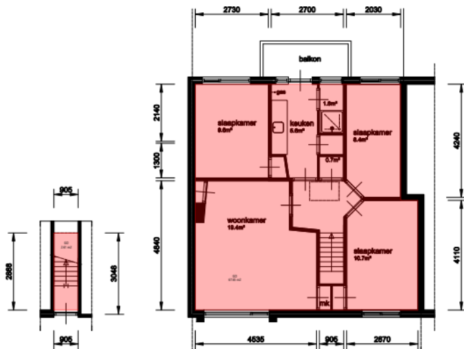
Verdieping
