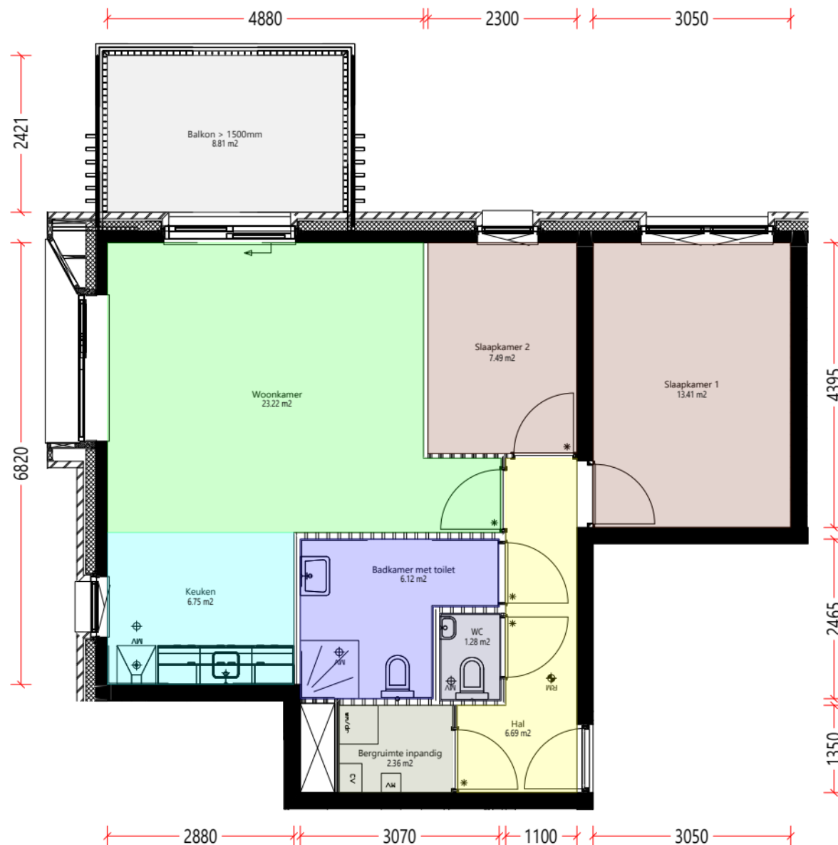
Verdieping_3e
