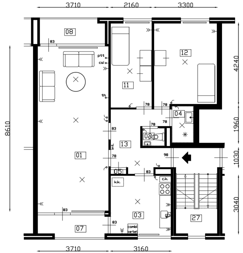
PLATTEGROND
