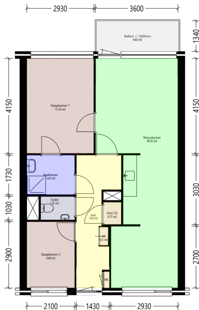
Verdieping_1e
