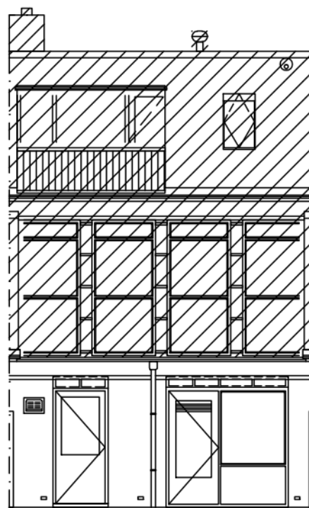
Achtergevel
