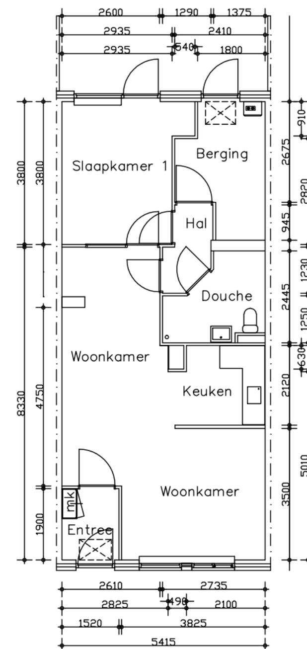
Beganegrond
