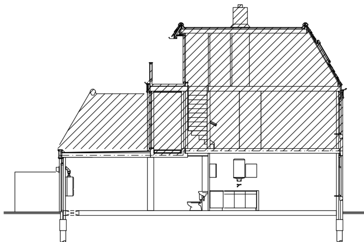
Doorsnede
