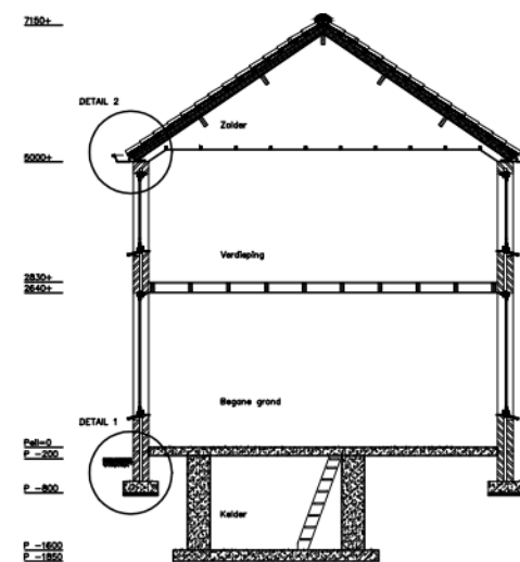
DOORSNEDE A-A
