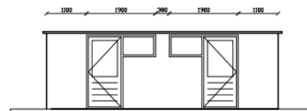
VOORGEVEL
