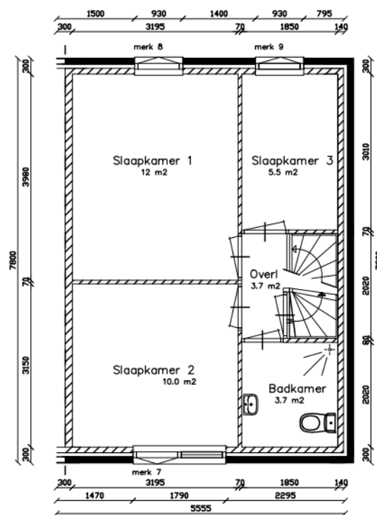
Verdieping
