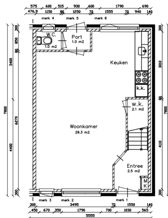
Begane grond
