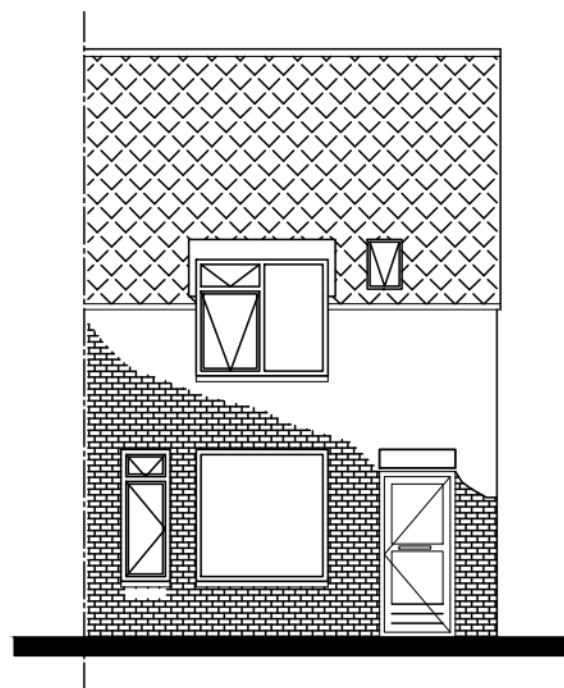
Voorgevel
