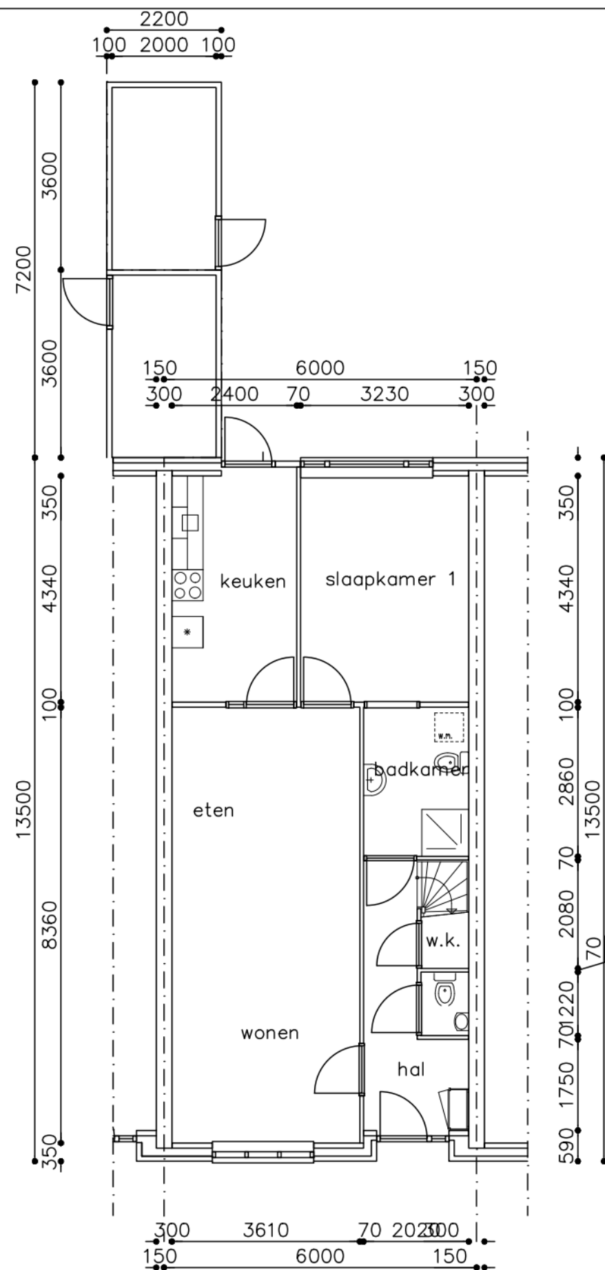
begane grond
