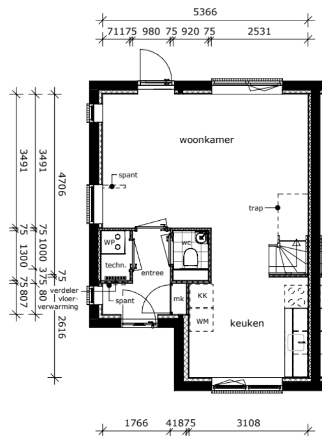
Begane grond 1 : 100
