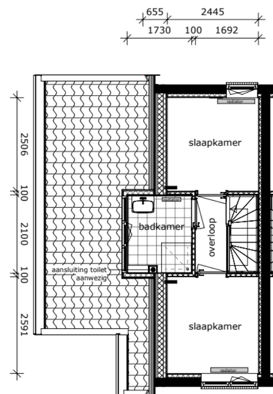
1e Verdieping 1 : 100
