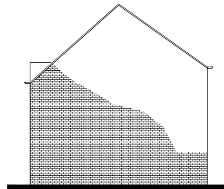
Zijgevel
