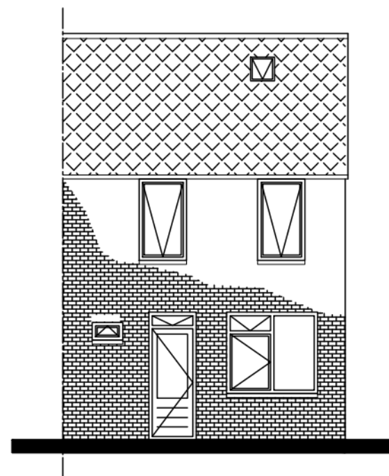
Achtergevel
