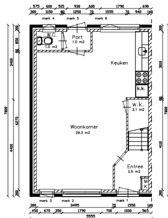
Beganegrond
