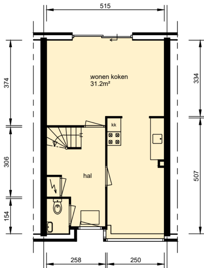
begane grond
