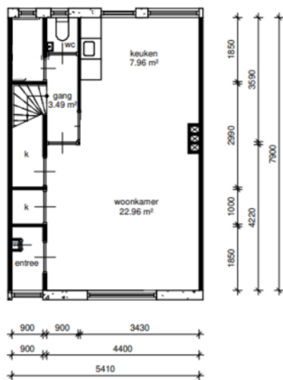
begane grond
