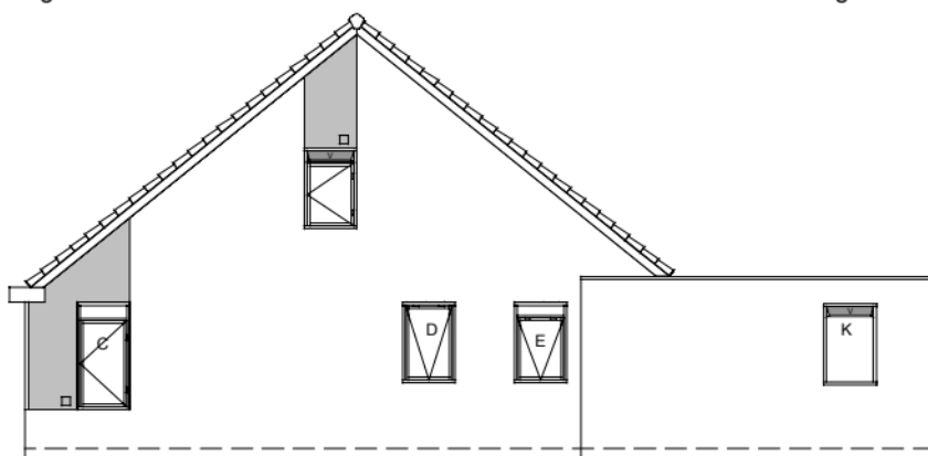
Eindgevel
