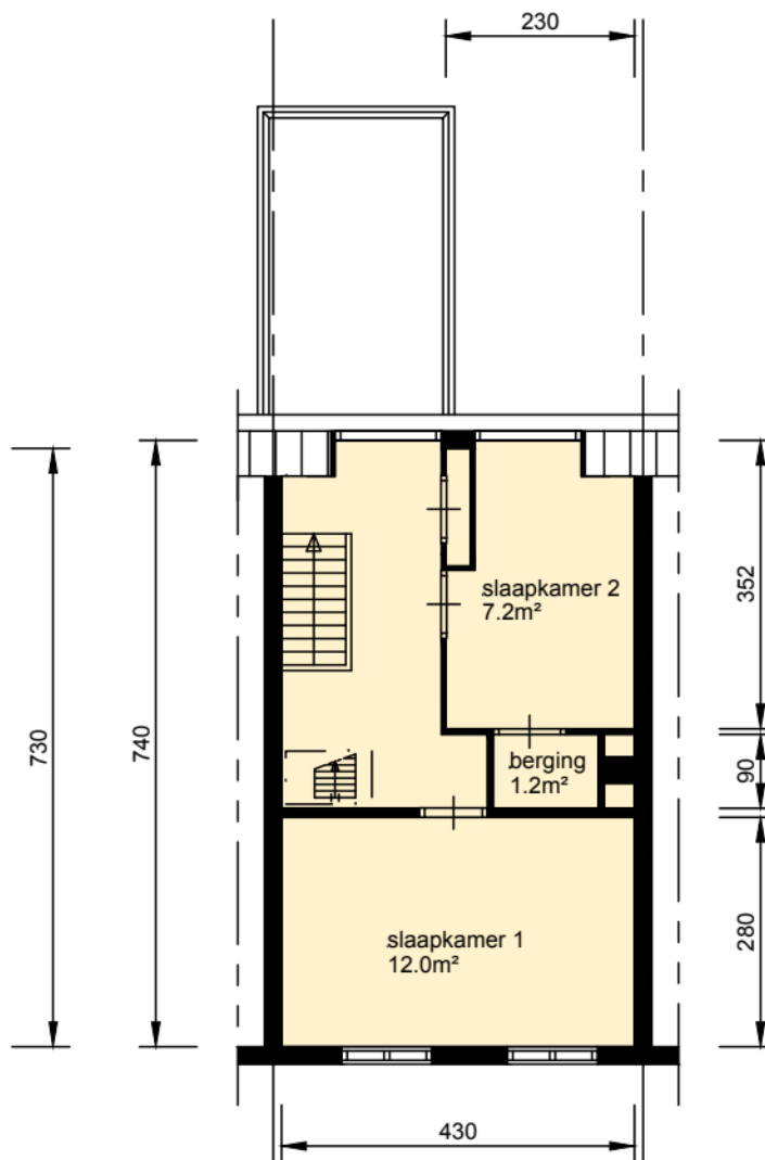
verdieping
