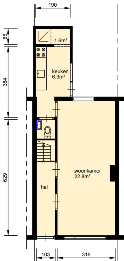
begane grond
