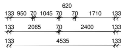
begane grond
