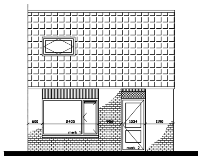
Voorgevel
