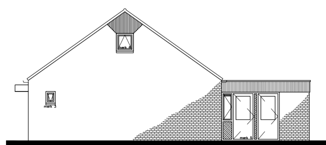
Rechterzijgevel
