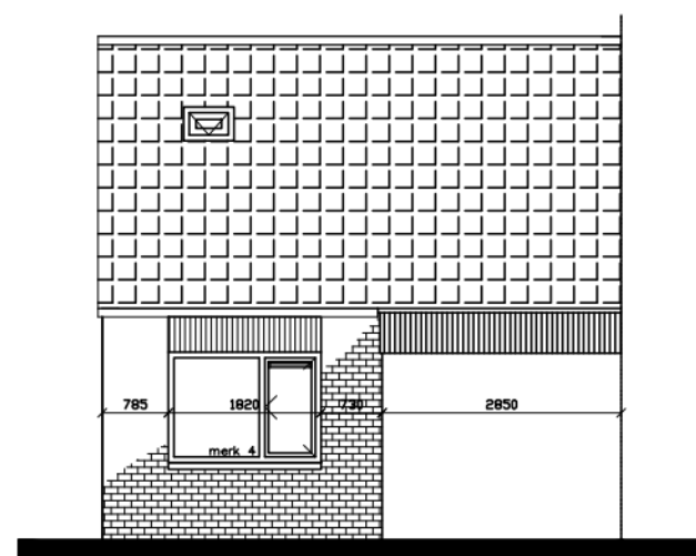
Achtergevel
