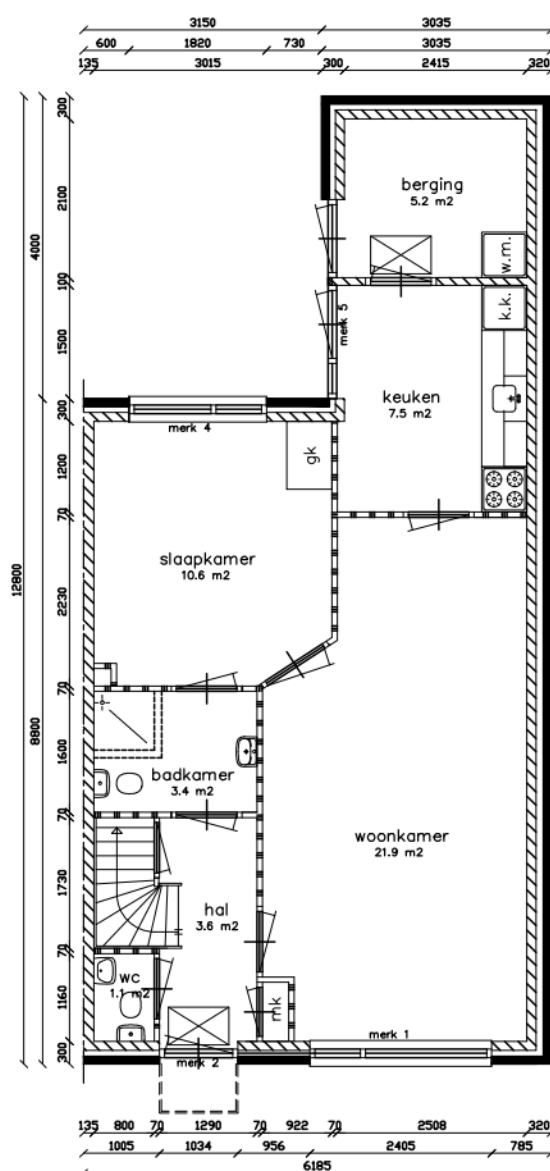
Begane grond
