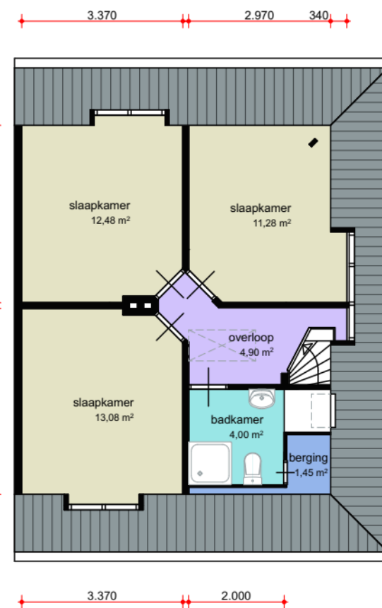
1ste Verdieping
