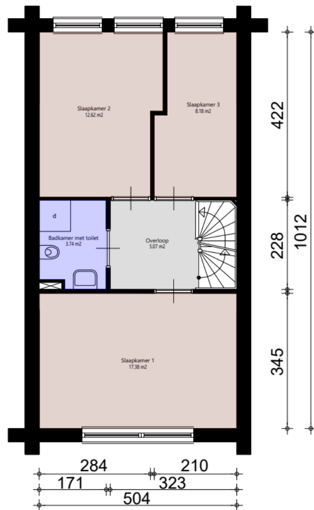
Verdieping_1e
