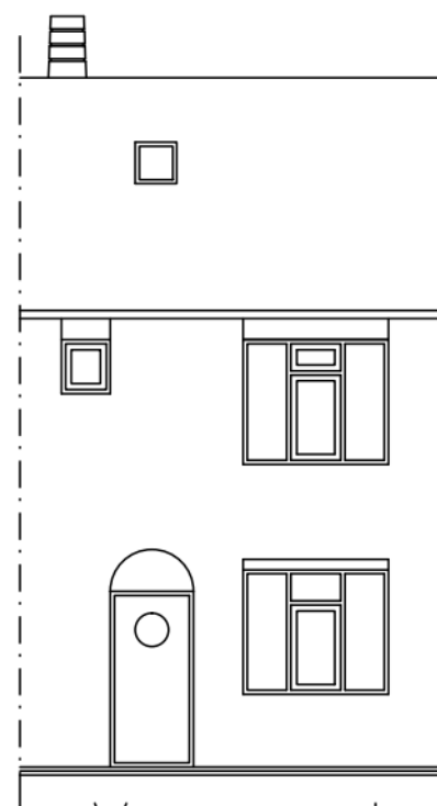
Voorgevel
