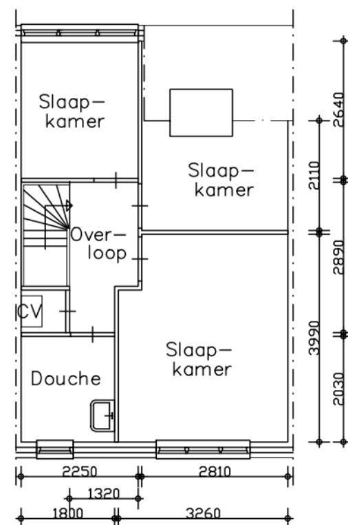
Verdieping
