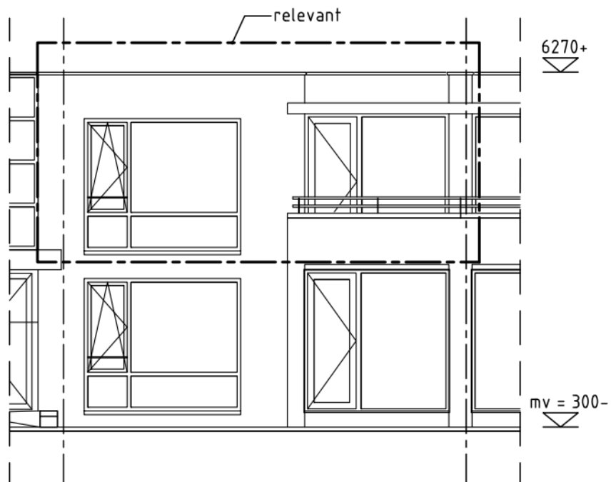
Achtergevel
