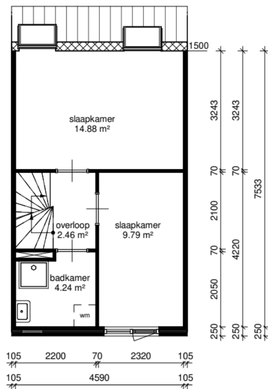
eerste verdieping
