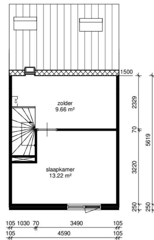
tweede verdieping
