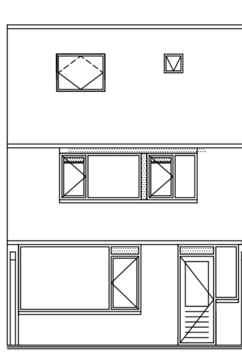
Achtergevel
