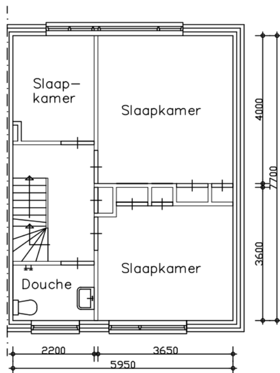
Verdieping
