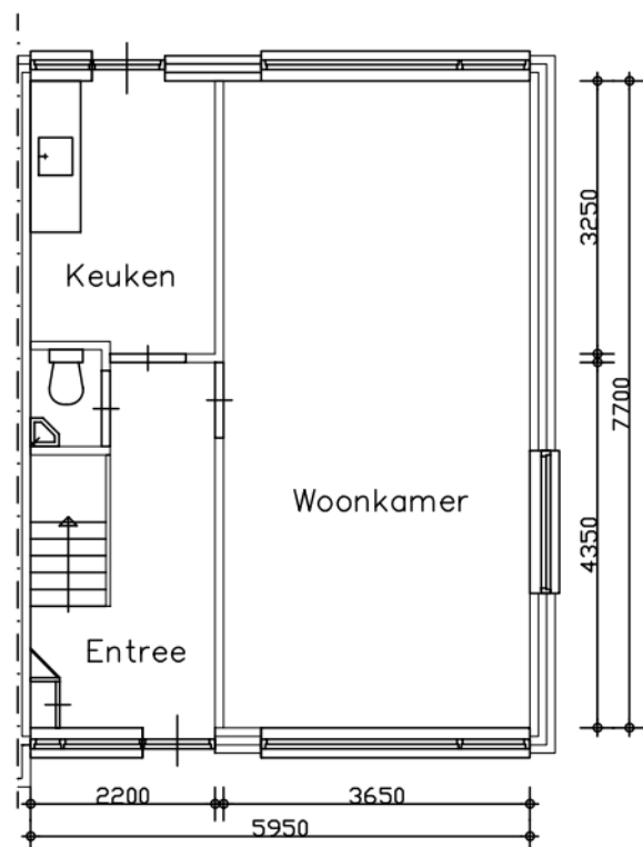
Begane grond
