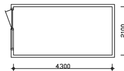
Plattegrond Berging
