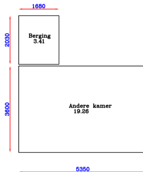
1e Verdieping
