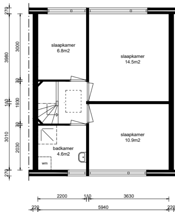
1e verdieping
