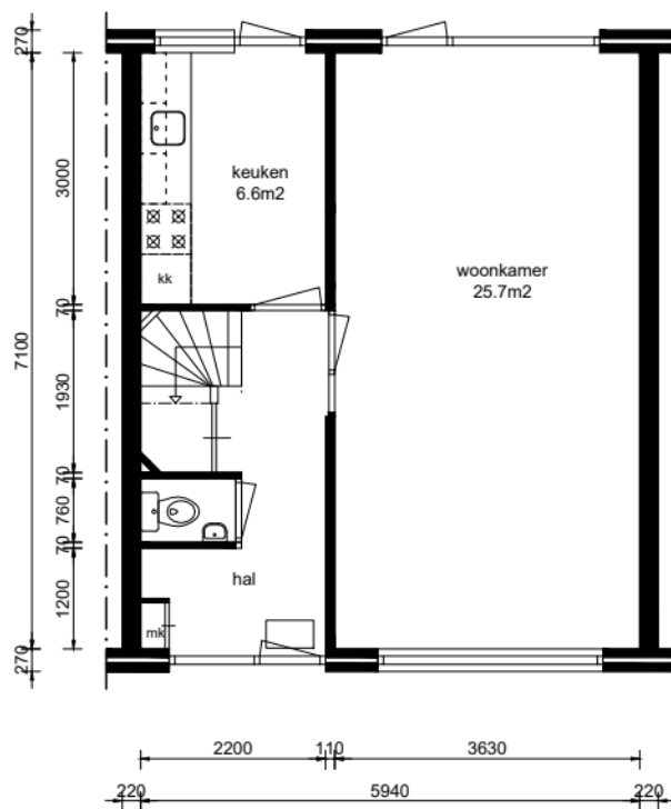
begane grond
