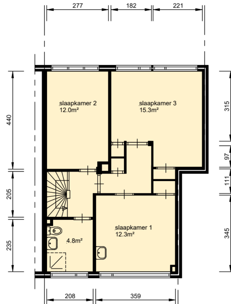
verdieping
