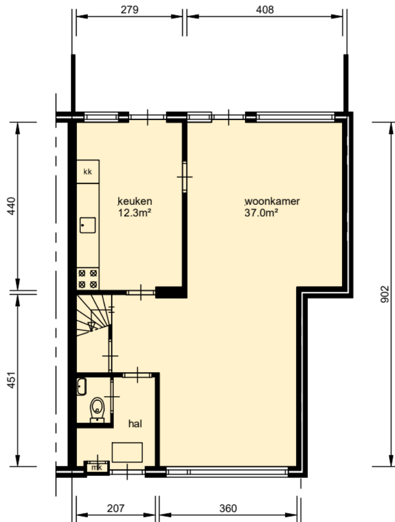
begane grond
