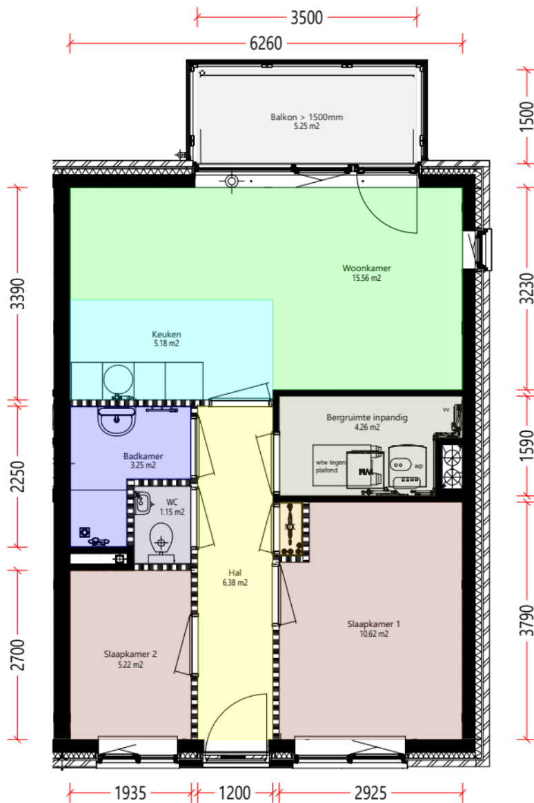
Verdieping_3e
