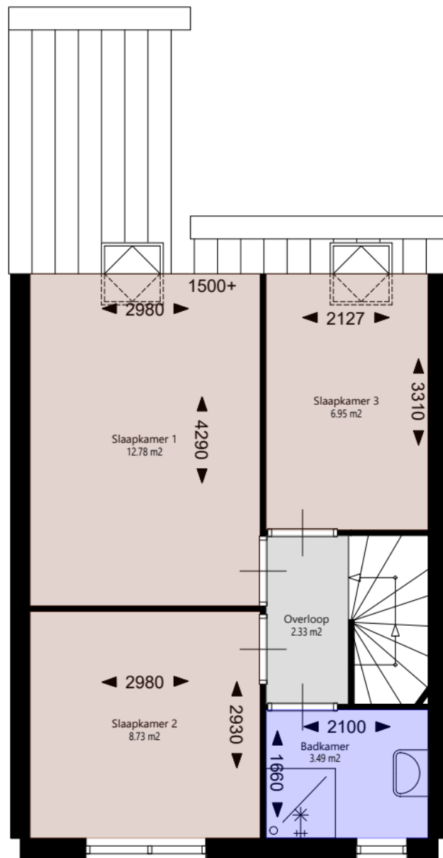
Verdieping_1e
