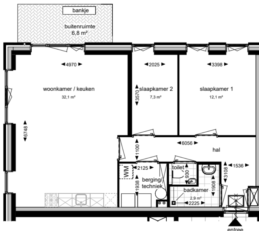
begane grond
