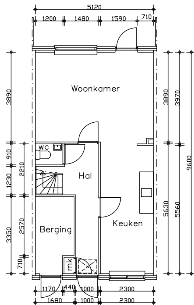
Begane grond
