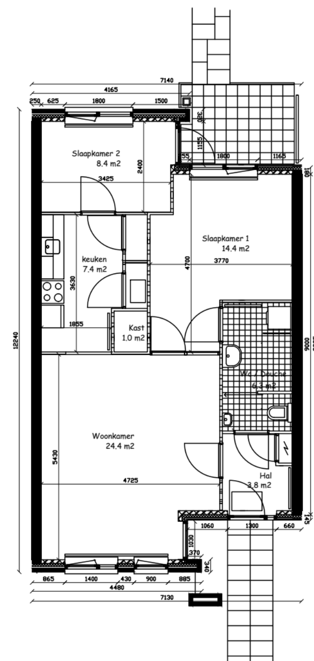
Begane grond
