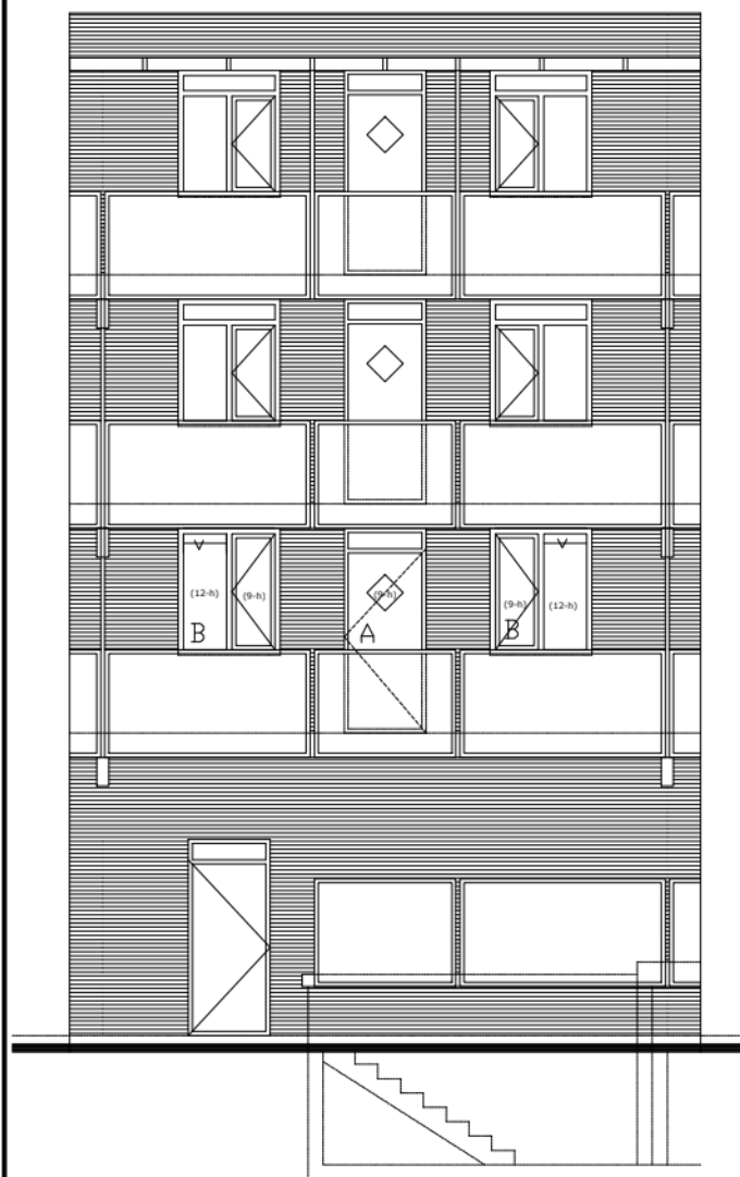
VOORGEVEL
