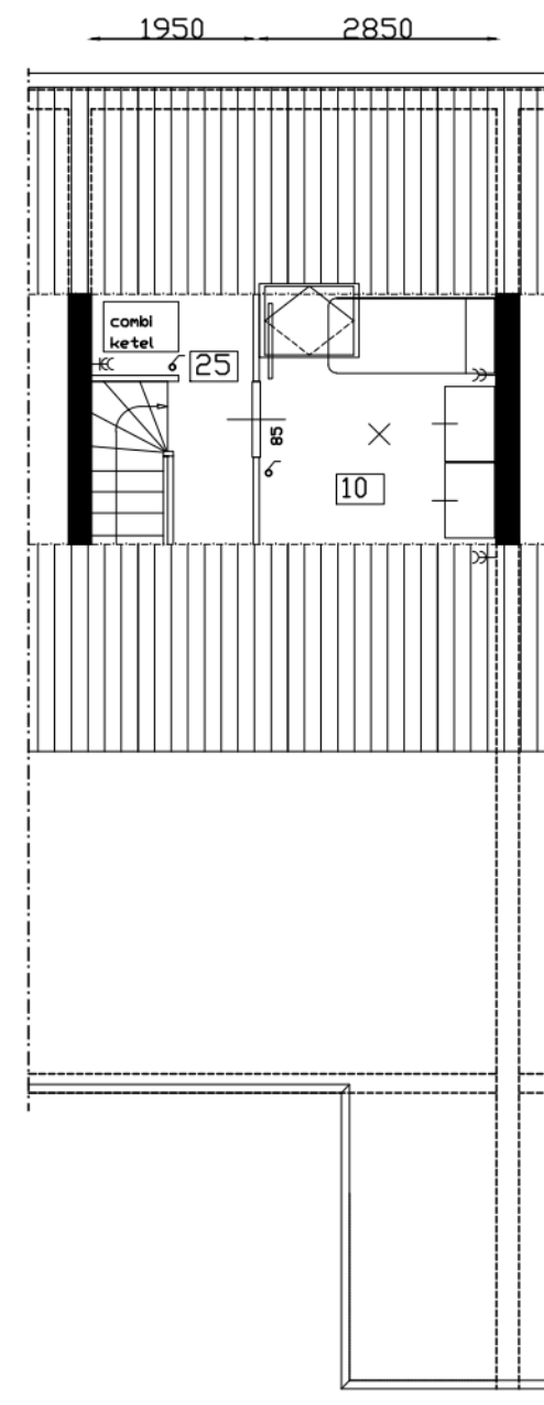
VERDIEPING
