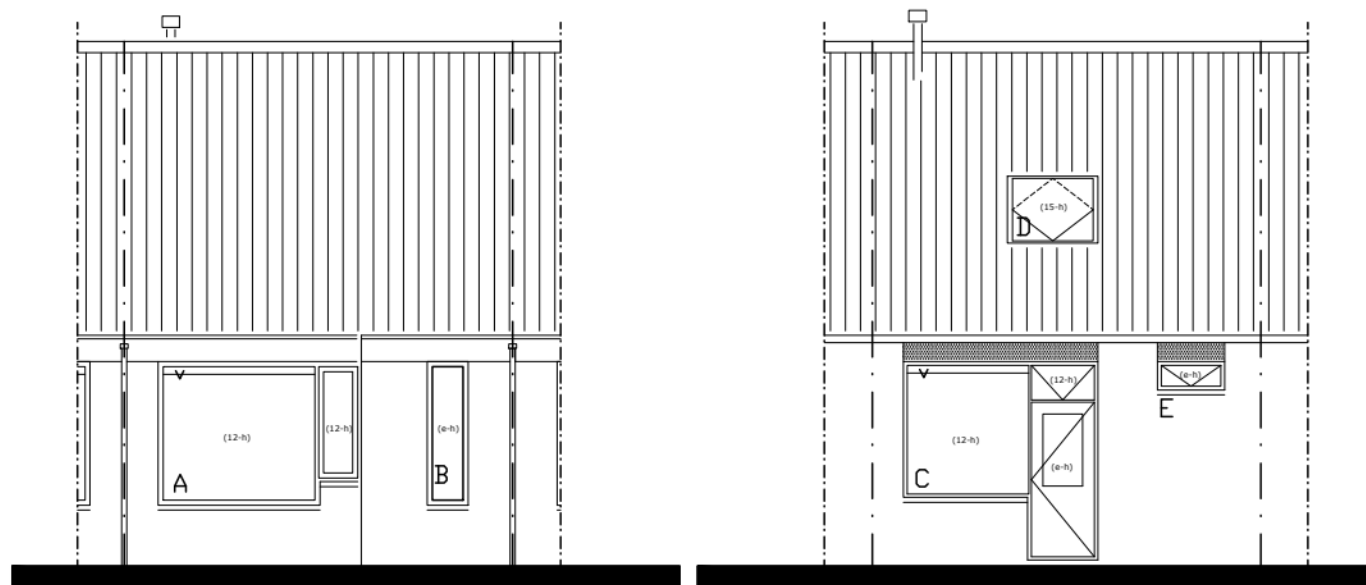
VOORGEVEL
