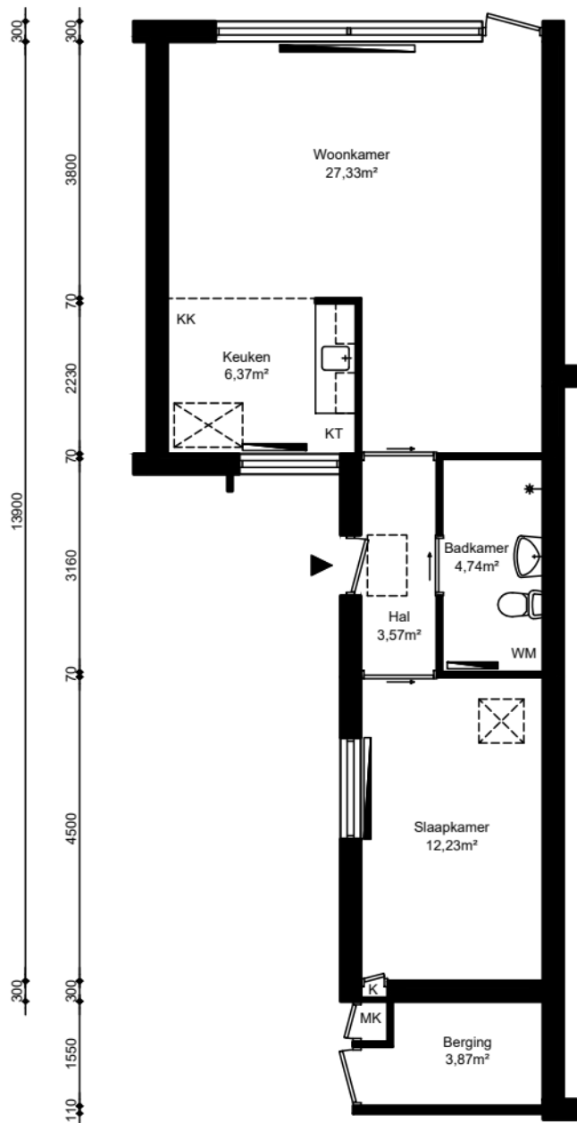
Begane grond
