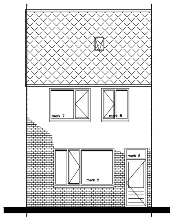
Achtergevel
