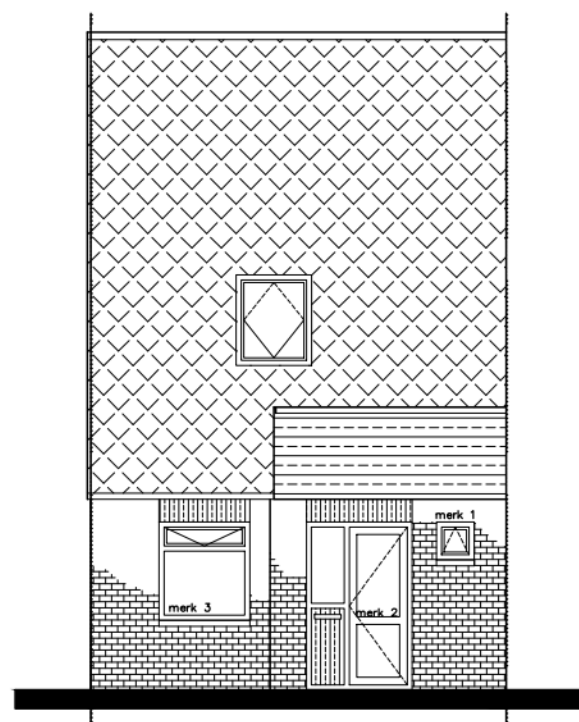
Voorgevel
