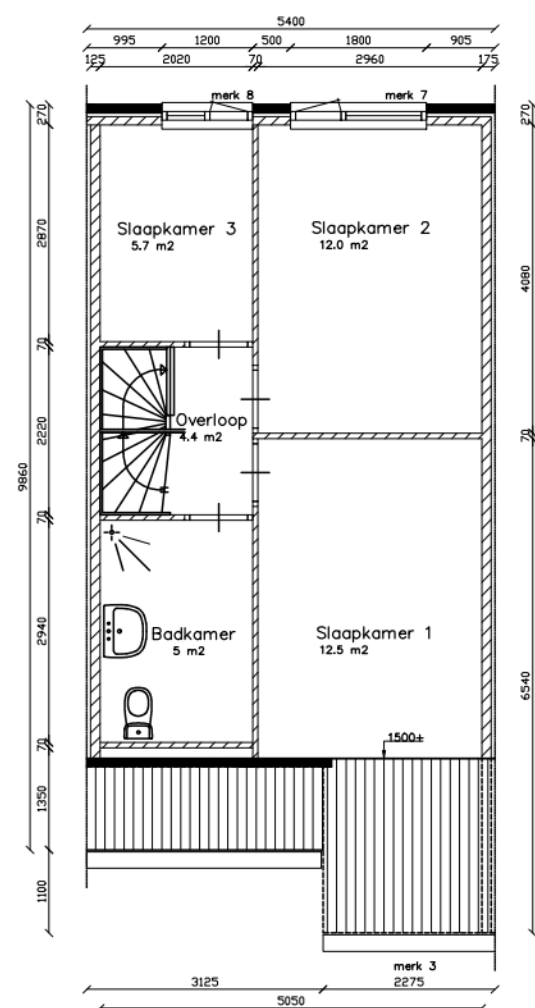
Verdieping
