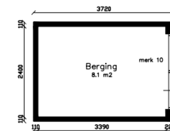
Platte-grond
