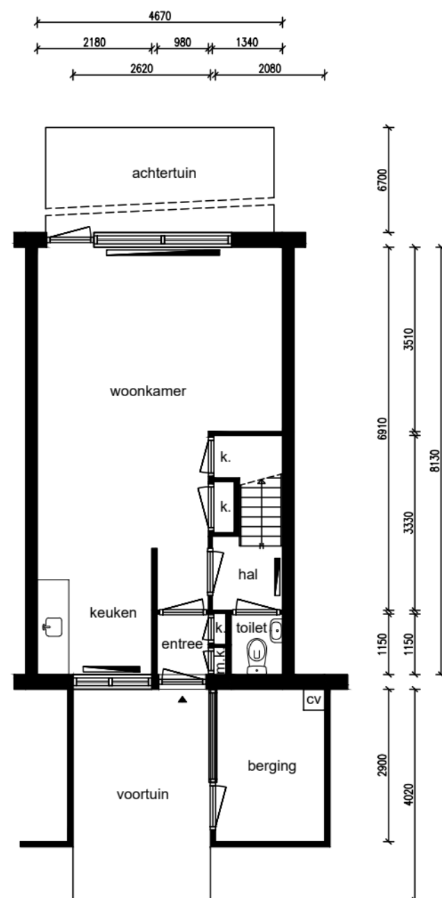
Begane grond
