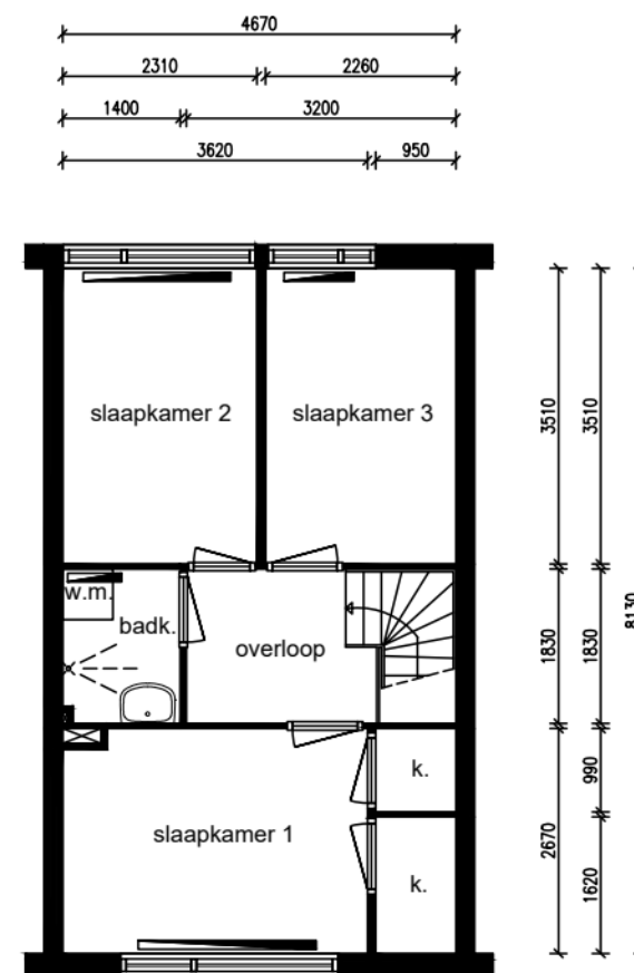
1e verdieping
