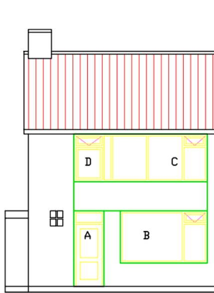
Voorgevel
