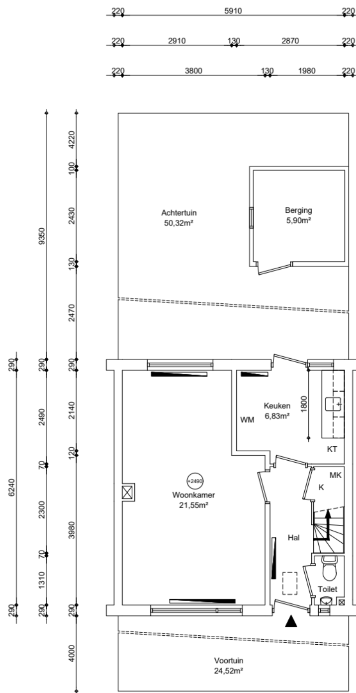
Begane grond GO wonen 36,88m²
