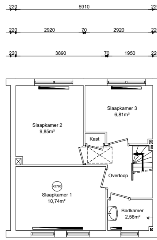
1e verdieping GO wonen 36,88m²
