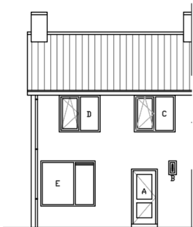
Voorgevel
