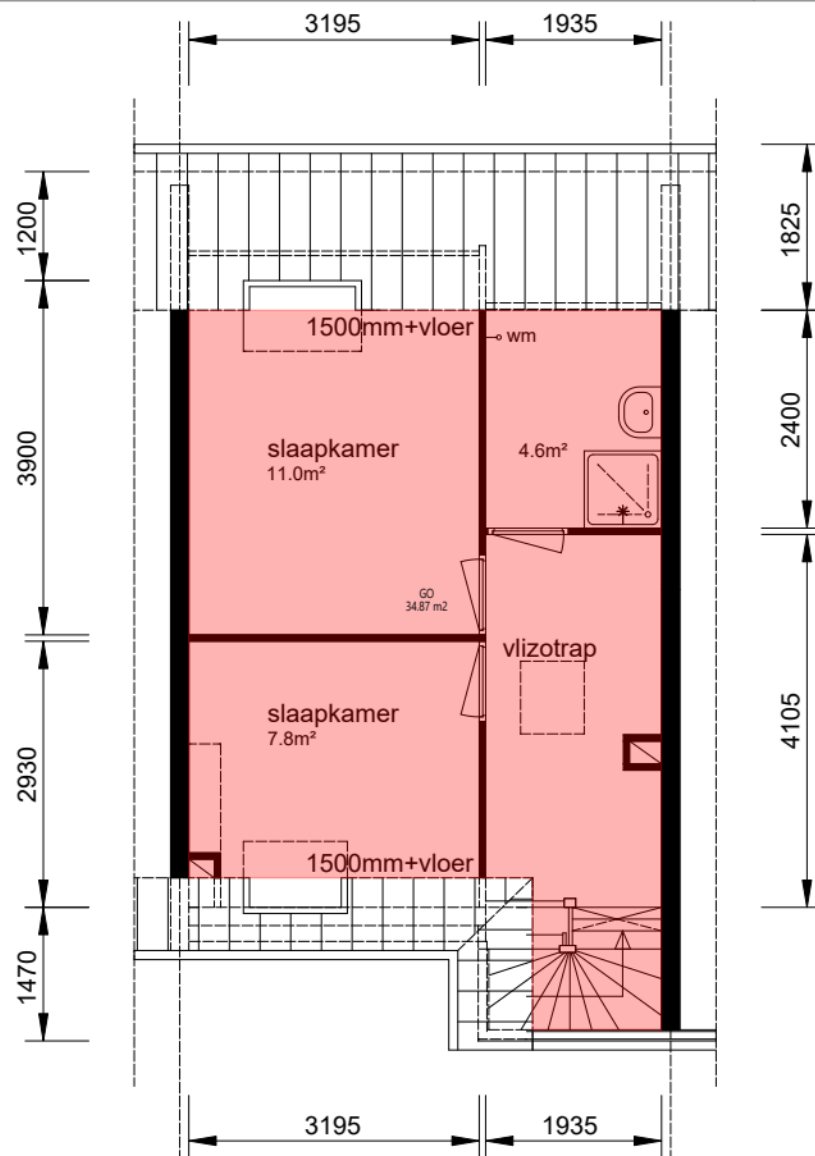
Verdieping_1e
