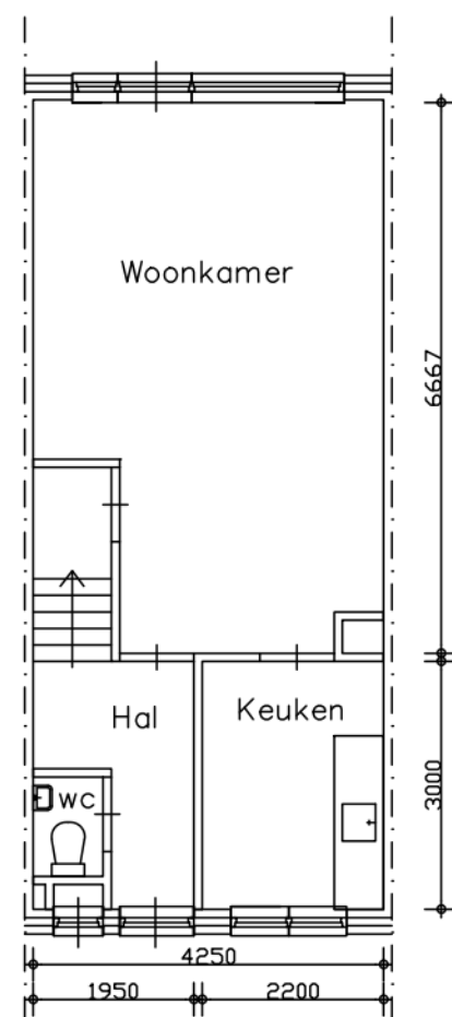
Begane grond
