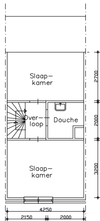
Verdieping
