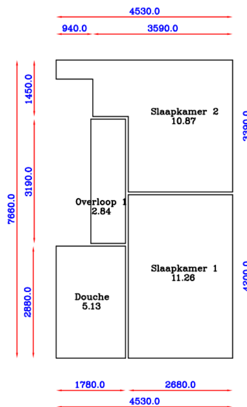
1e Verdieping
